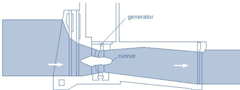
Turbina de maré 'Stratflow'
